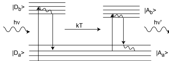
Figure 6: Energy diagram for Förster transfer
