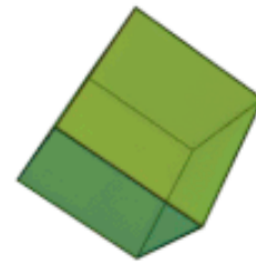
Würfel – Erde
