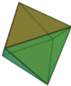
Oktaeder – Luft
