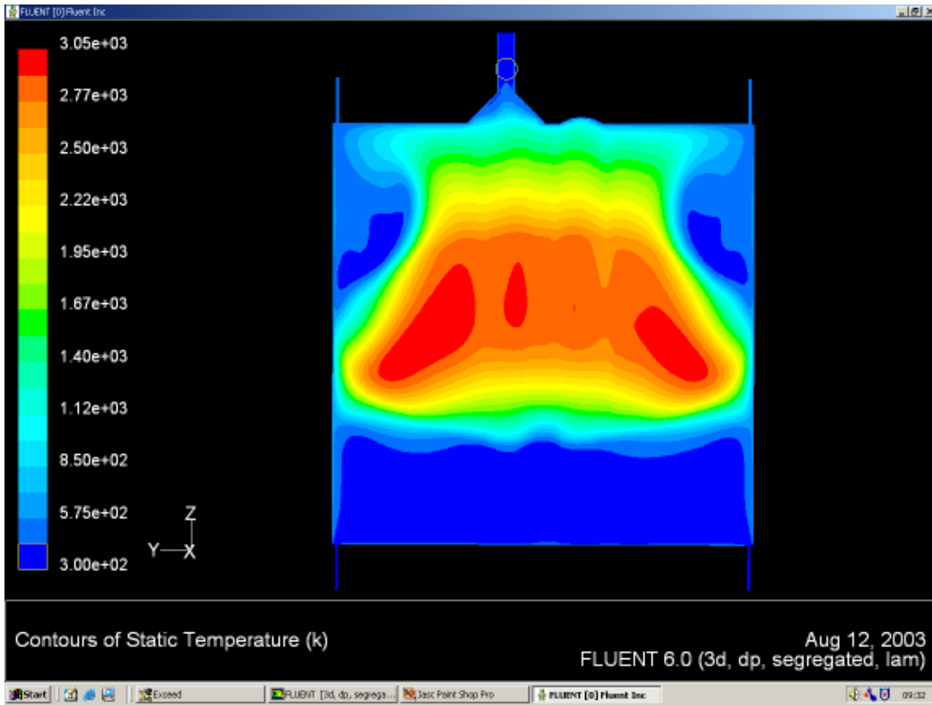
Temperaturverteilung
